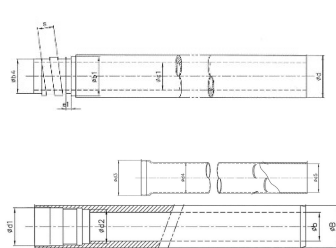
ボーリングバー 機械的強度の大きな特殊鋼を使用し熱処理を行い、高い剛性とトルクに耐えられる特殊設計
