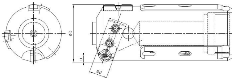
CR型（レンチ型）
