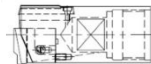
組立式特殊2段刃ヘッド
