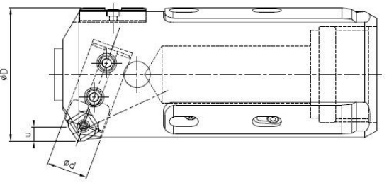
CR型 (レンチ型)
