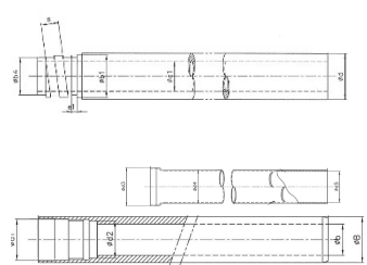
ボーリングバー 機械的強度の大きな特殊鋼を使用し熱処理を行い、高い剛性とトルクに耐えられる特殊設計
